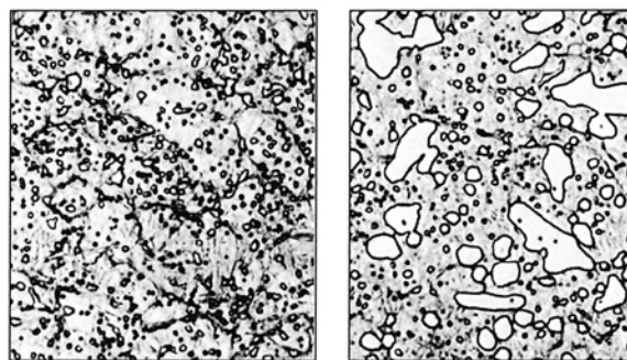
Rigor (ASSAB XW-10) とAISI D3 (SKD1) 相当の高カーボン、高クロム鋼とのマイクロ組織の比較
